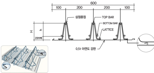
SPEED DECK 단면상세도
