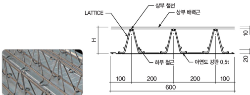
TG DECK PLATE 단면상세도
