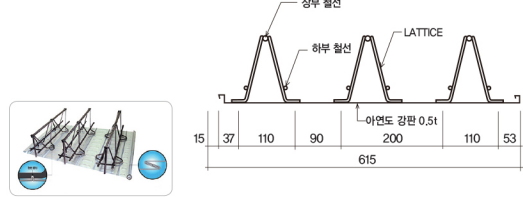
NT DECK PLATE 단면상세도
