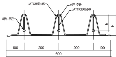
ECONO DECK PLATE 단면상세도
