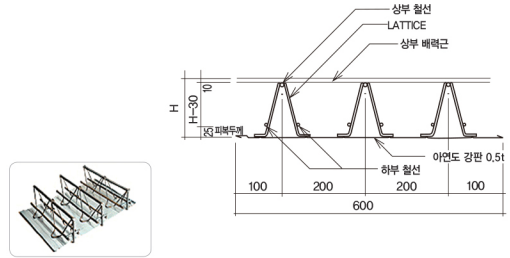
TRUSS DECK PLATE 단면상세도
