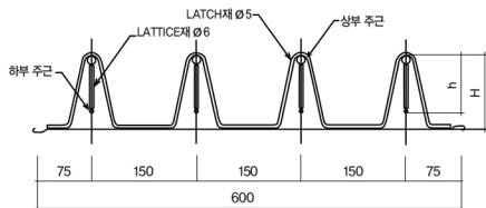
FERRO DECK PLATE 단면상세도
