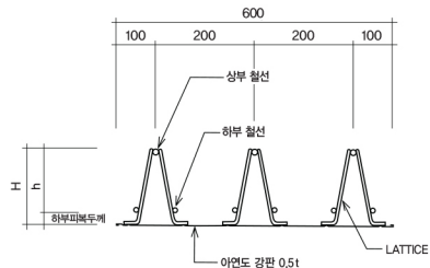
SUPER DECK PLATE-T TYPE 단면 상세도
